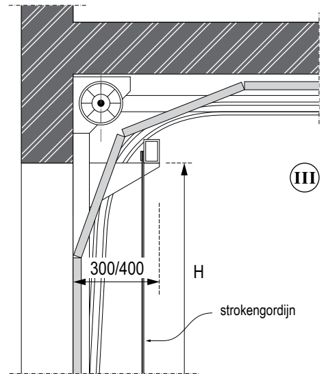
verticale doorsnede
