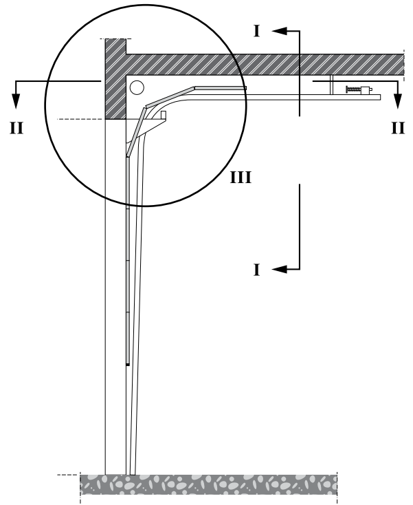
verticale doorsnede
