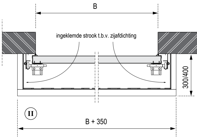
horizontale doorsnede
