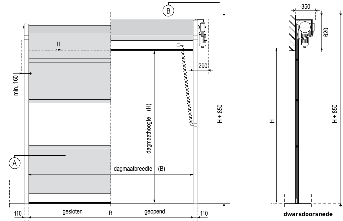
vooraanzicht
