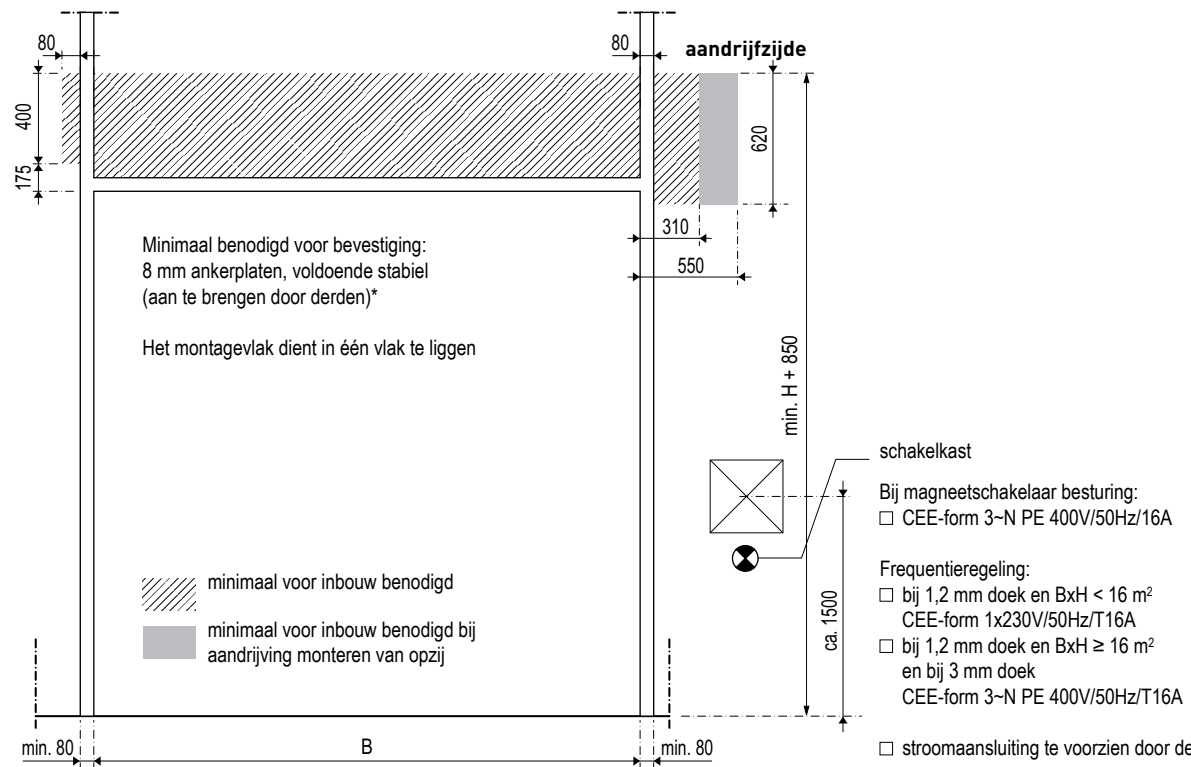
bouwkundige voorzieningen
